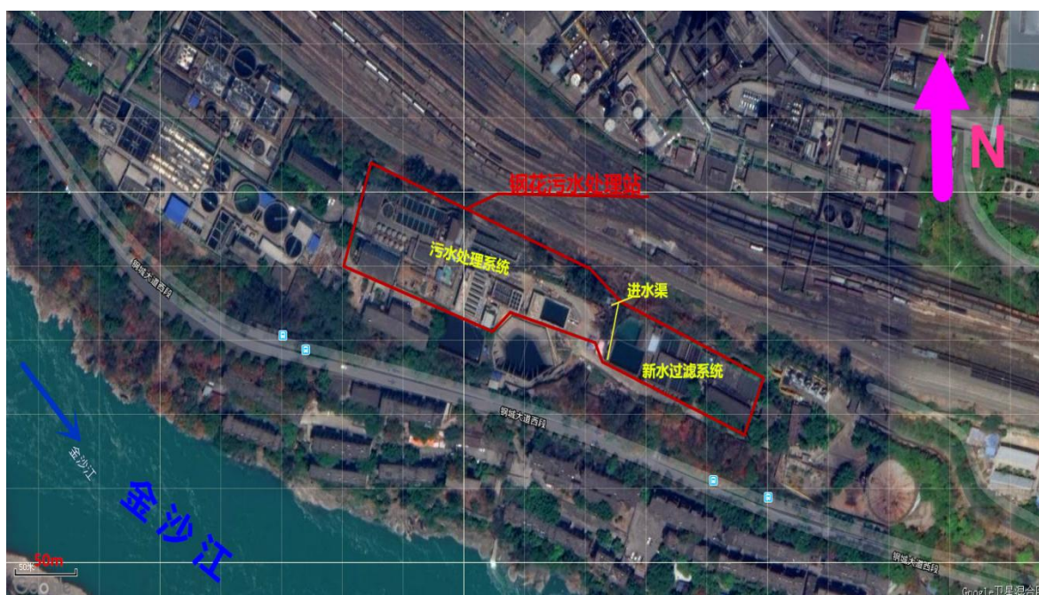
图 4.2-4 钢花污水处理站平面布置图
