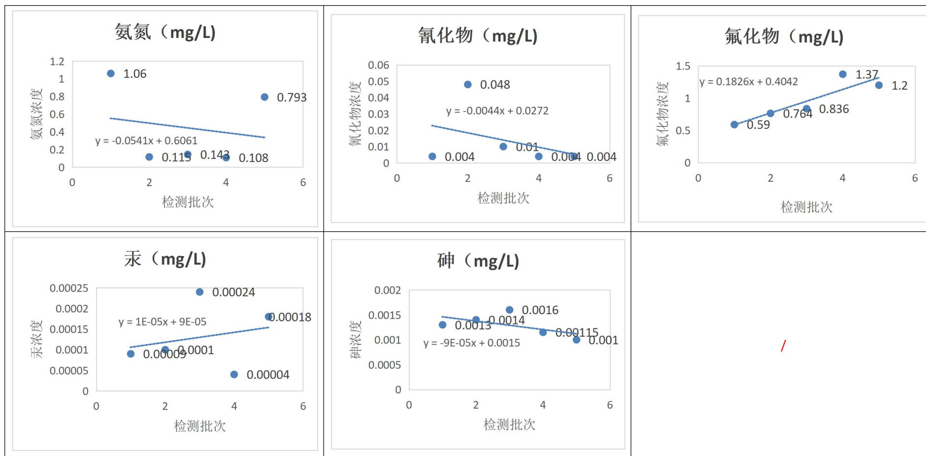
图 8.2-2 AS2 监测井污染物浓度监测值变化及趋势预测
