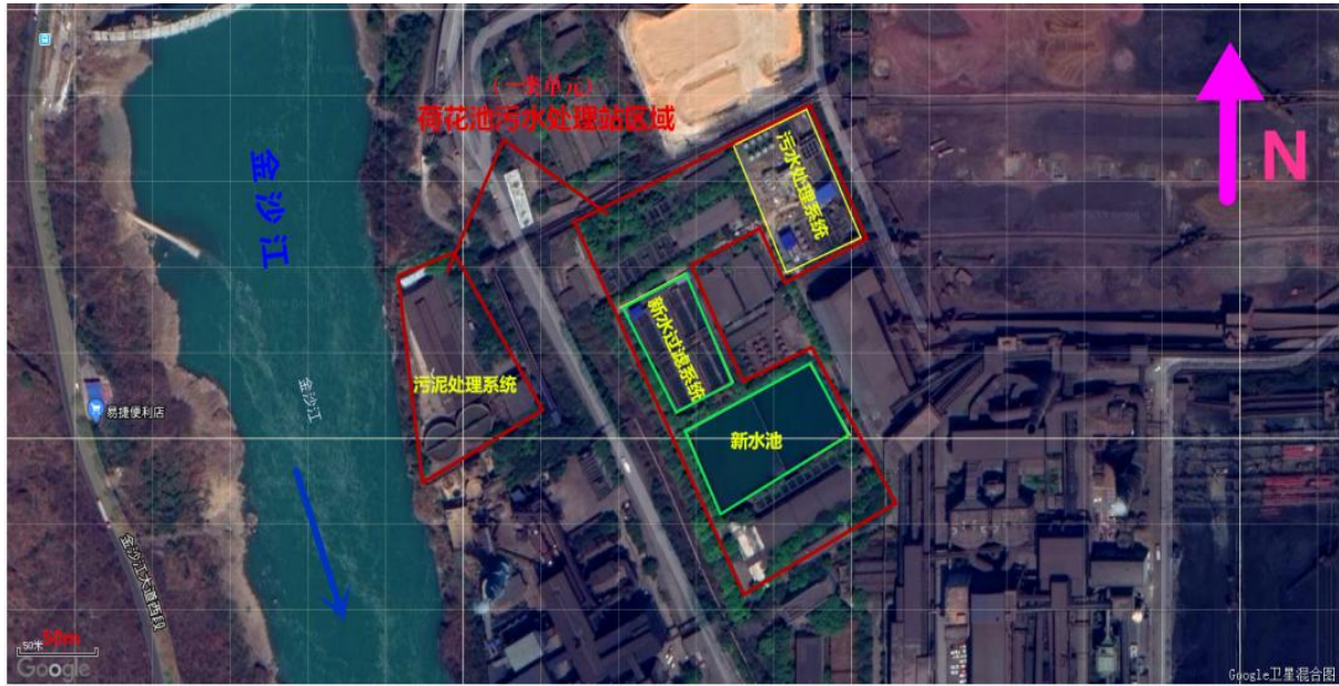
图 5.1-3 荷花池污水处理站重点监测单元分布图
