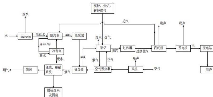
图 4.1-13 热电系统工艺流程
