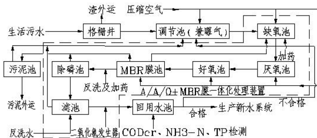
图 4.1-11 西部生活污水处理工艺流程图
