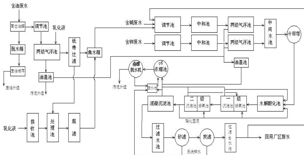
图 4.1-6 含锌、含碱、含油废水处理工艺流程图
