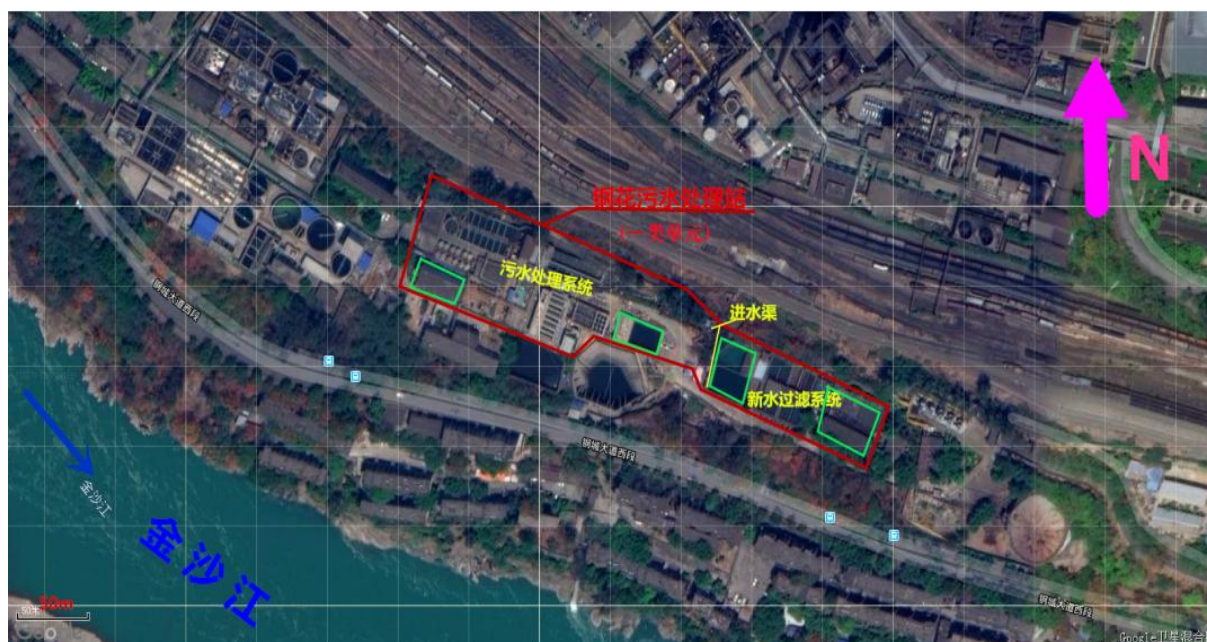
图 5.1-2 钢花污水处理站重点监测单元分布图
