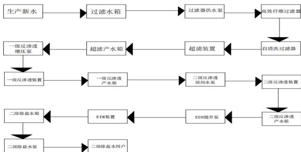
图 4.1-14 除盐水工艺流程图
