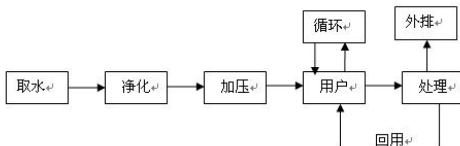
图 4.1-1 能源动力分公司给水系统总体工艺流程图
