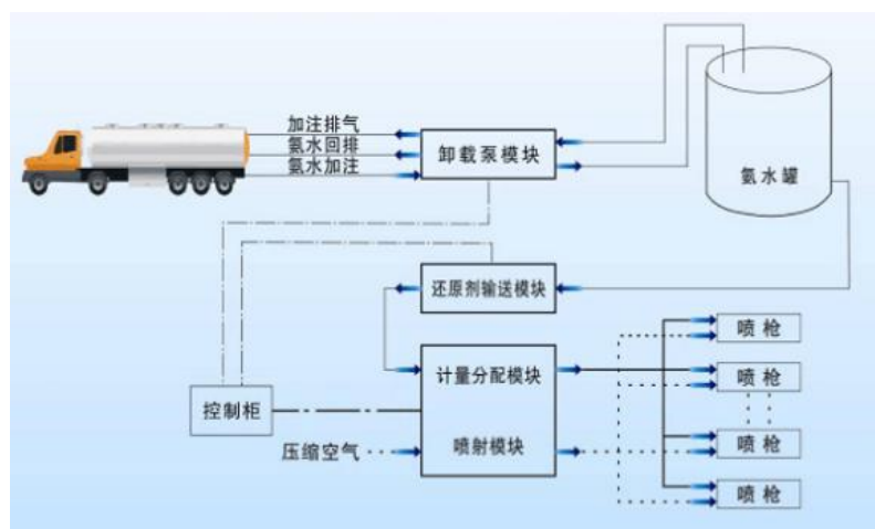
图 4.1-16 SCR 系统工艺流程简图
