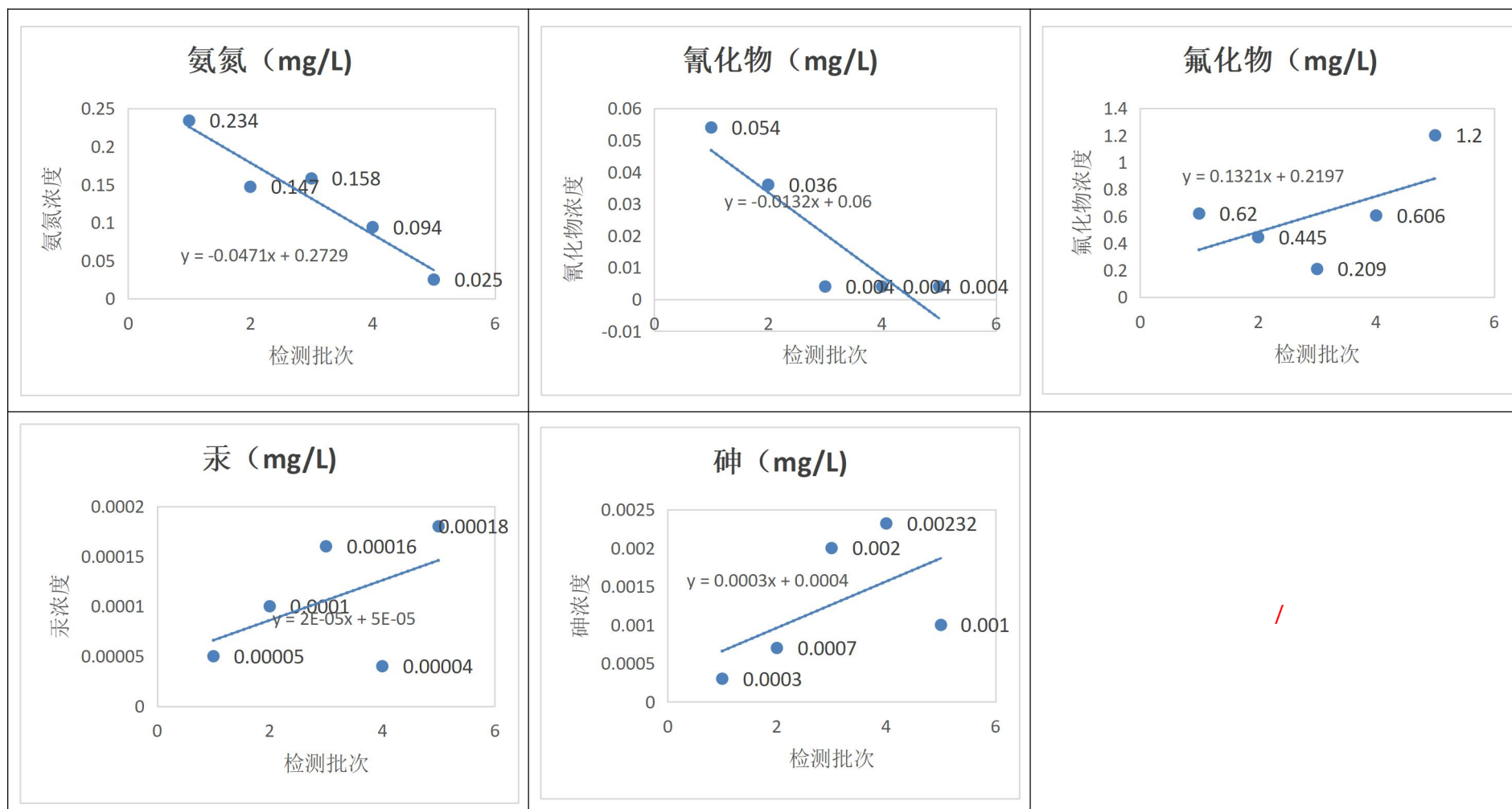
图 8.2-1 AS1 监测井污染物浓度监测值变化及趋势预测
