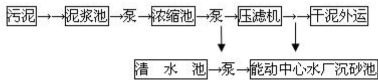
图 4.1-9 污泥处理站工艺流程图
