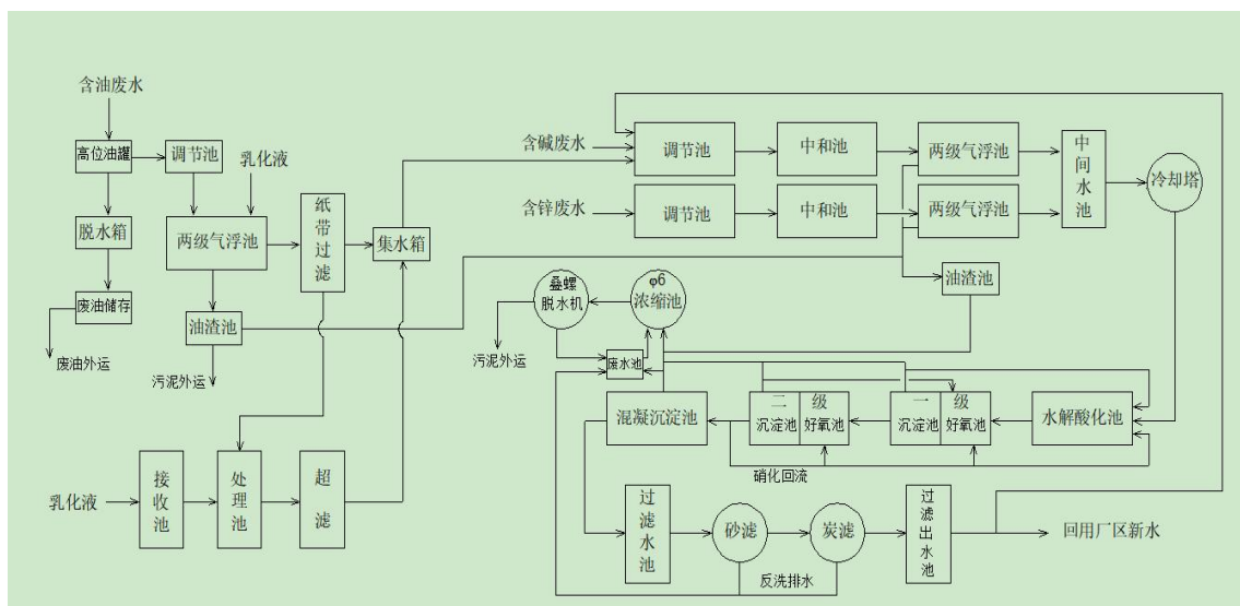
图 4.1-5 酸性废水处理工艺图
