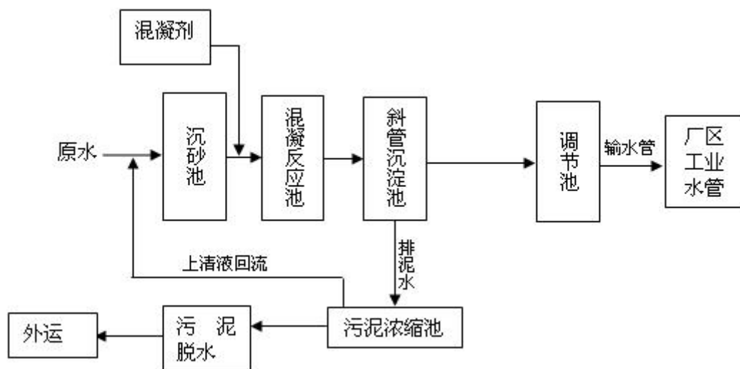
图 4.1-2 取水净化工艺流程图
