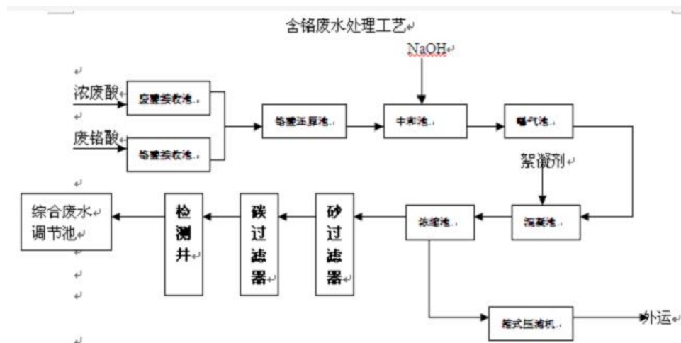
图 4.1-7 冷轧废铬酸处理工艺流程图
