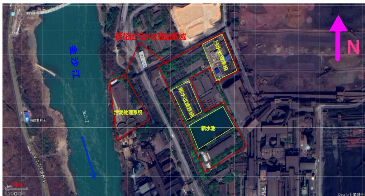
图 4.2-3 荷花池污水处理站平面布置图
