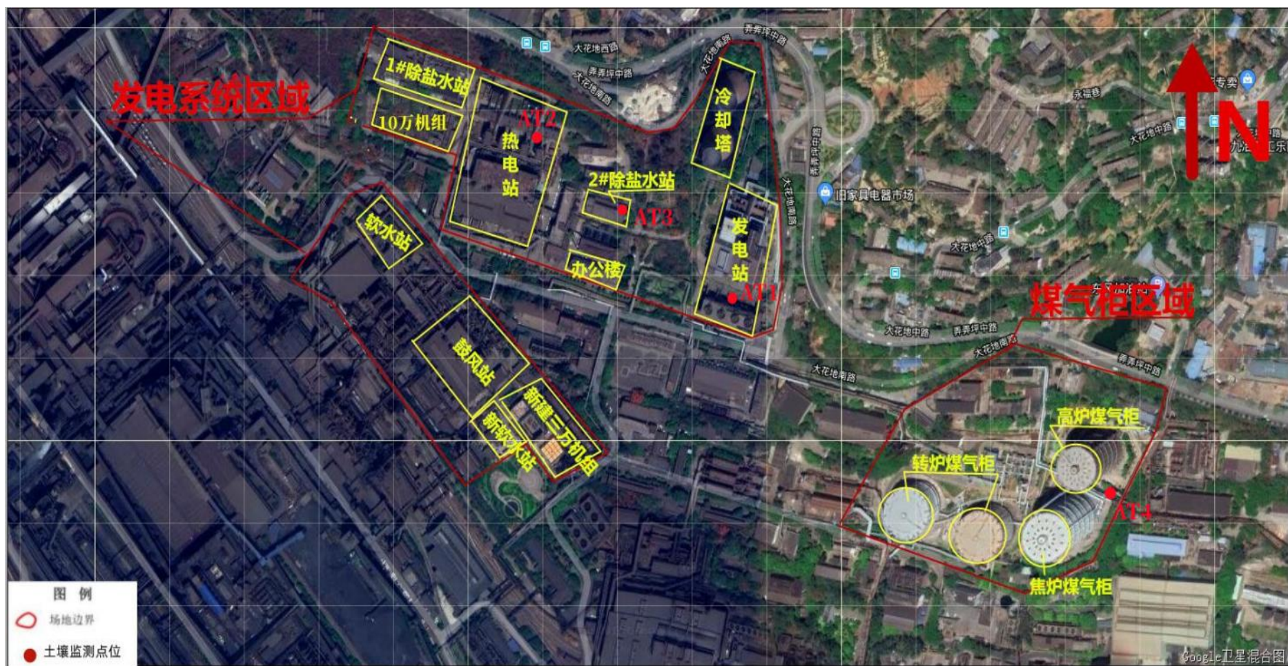
图 6.3-1 能源动力分公司发电系统、煤气柜系统区域土壤监测点位示意图
