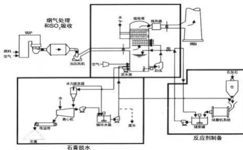
图 4.1-15 石灰石膏法脱硫工艺流程简图
