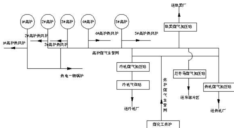
图 4.1-12 燃气系统煤气净化工艺流程图
